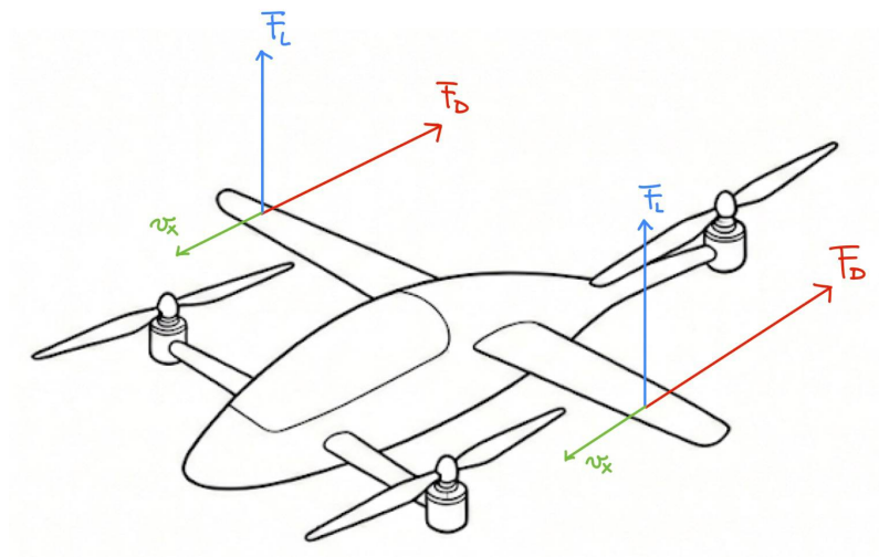
Figura 3.7: Portanza e Resistenza lungo l'asse X_b
