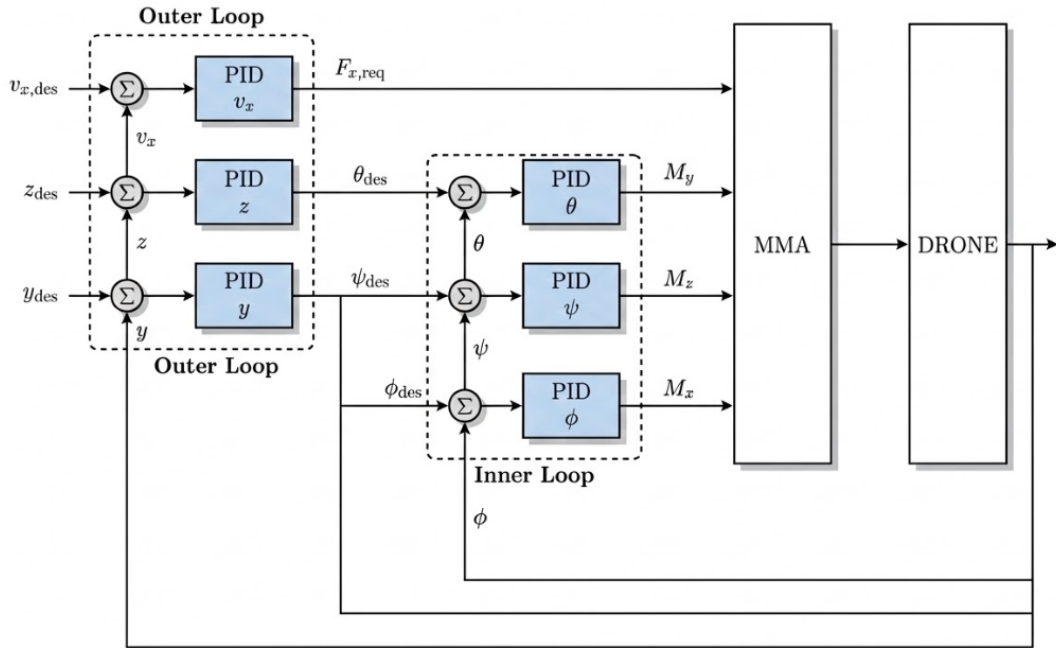
Figura 6.2: Schema a blocchi del controllo orizzontale.
