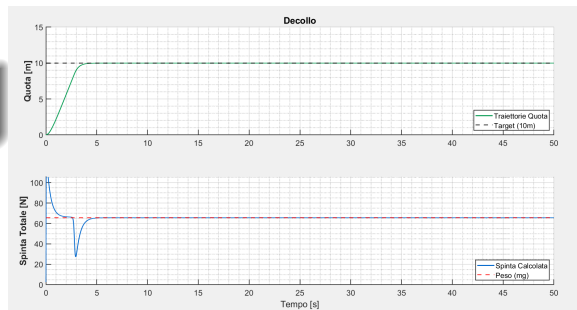
Figura 14: Tracking Quota e Spinta: Sovrapposizione di 100 simulazioni. Si nota il picco di spinta al lift-off e la successiva stabilizzazione al peso nominale.
