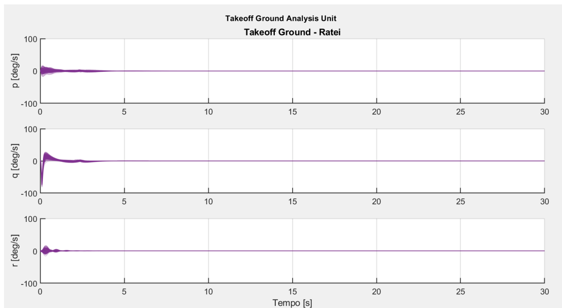
Figura 9.5: Evoluzione delle velocità angolari durante il takeoff.
