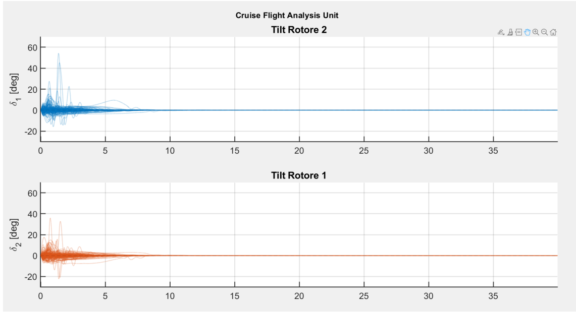
Figura 9.18: Evoluzione degli angoli di tilt dei rotori durante il volo traslato.
