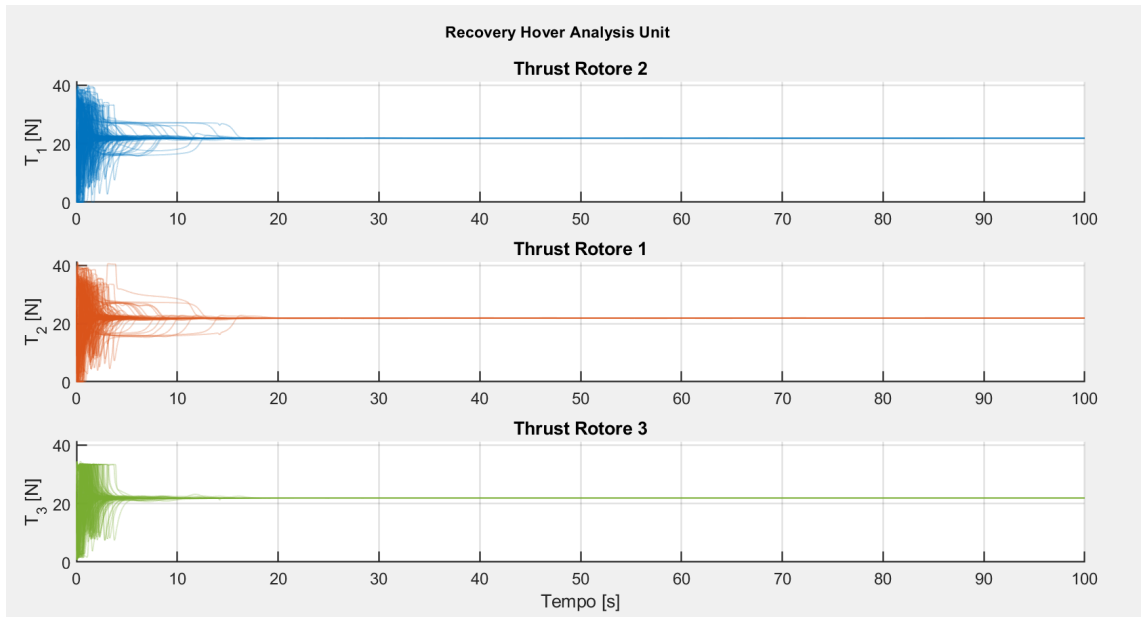
Figura 9.13: Evoluzione del thrust generato dai rotori in hovering.
