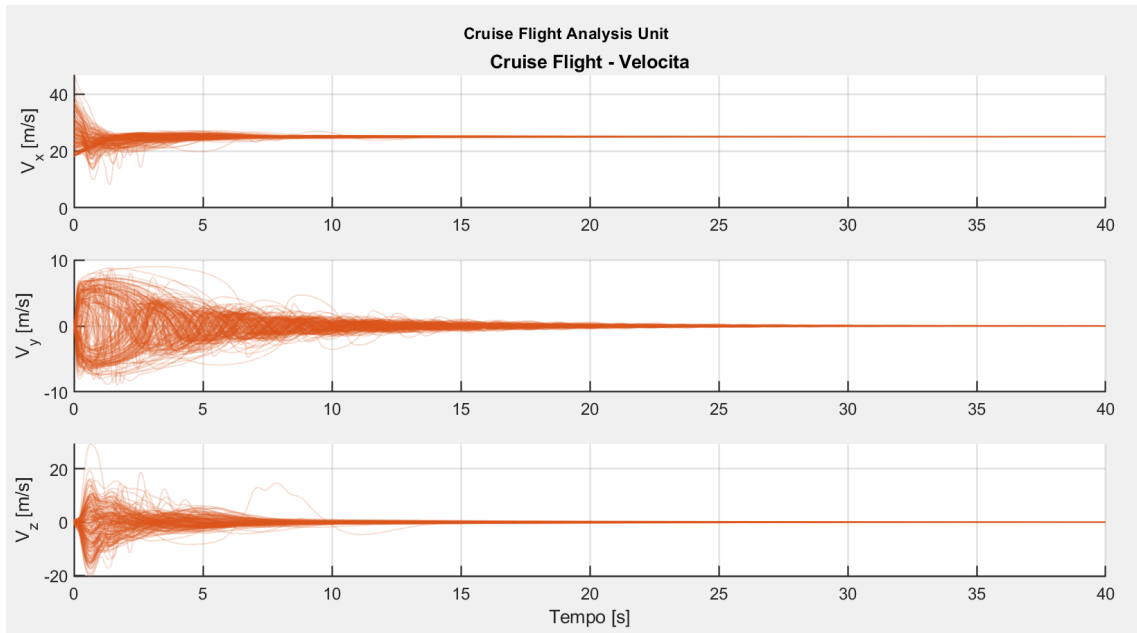
Figura 9.15: Evoluzione delle velocità lineari durante il volo traslato.
