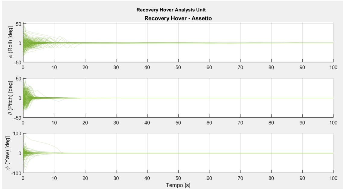
Figura 9.10: Evoluzione degli angoli di Eulero in hovering.
