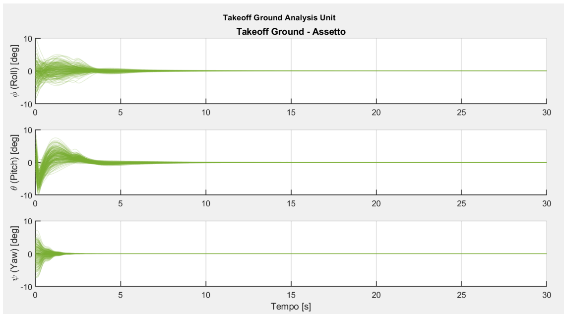
Figura 9.4: Evoluzione degli angoli di Eulero durante il takeoff.
