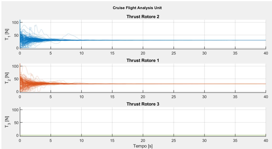
Figura 9.19: Evoluzione del thrust generato dai rotori durante il volo traslato.
