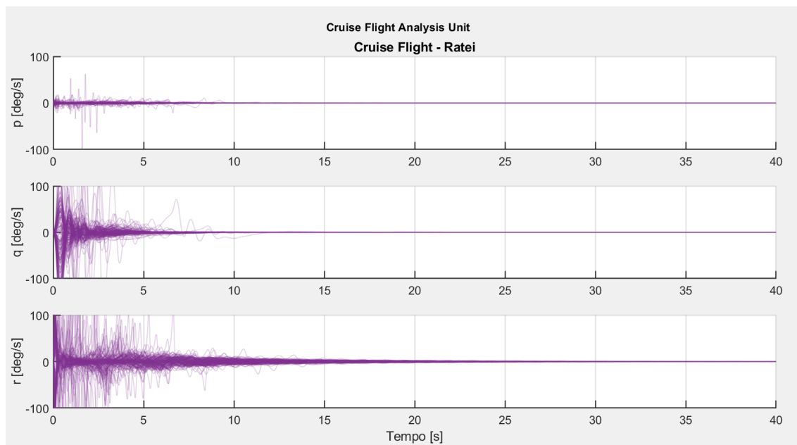
Figura 9.17: Evoluzione delle velocità angolari durante il volo traslato.
