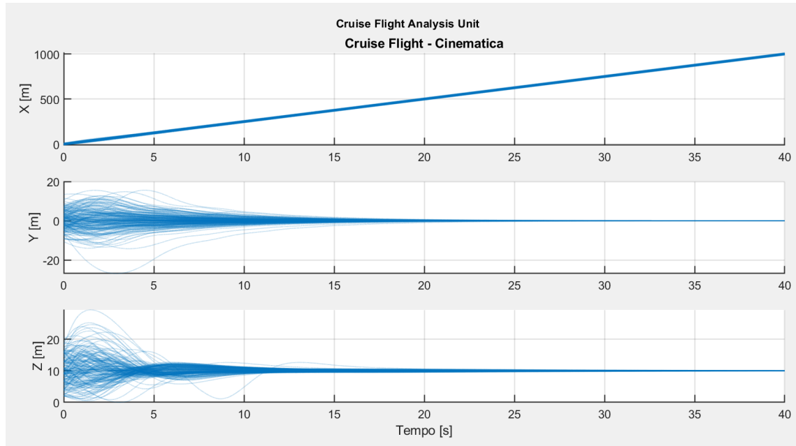
Figura 9.14: Evoluzione delle posizioni durante il volo traslato.
