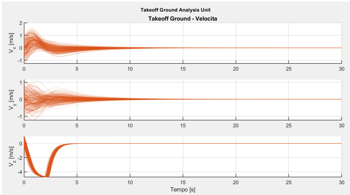
Figura 9.3: Evoluzione delle velocità lineari durante il takeoff.
