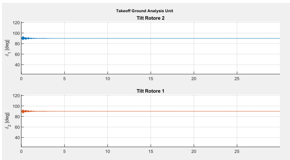
Figura 9.6: Evoluzione degli angoli di tilt dei rotori durante il takeoff.
