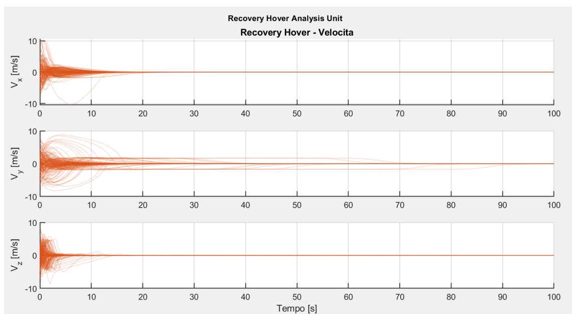
Figura 9.9: Evoluzione delle velocità lineari in hovering.
