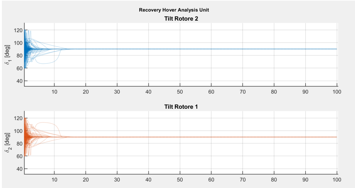
Figura 9.12: Evoluzione degli angoli di tilt dei rotori in hovering.
