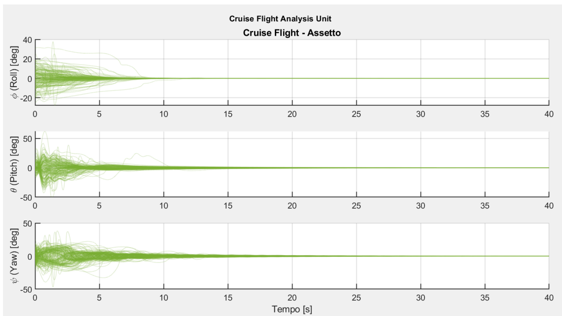
Figura 9.16: Evoluzione degli angoli di Eulero durante il volo traslato.
