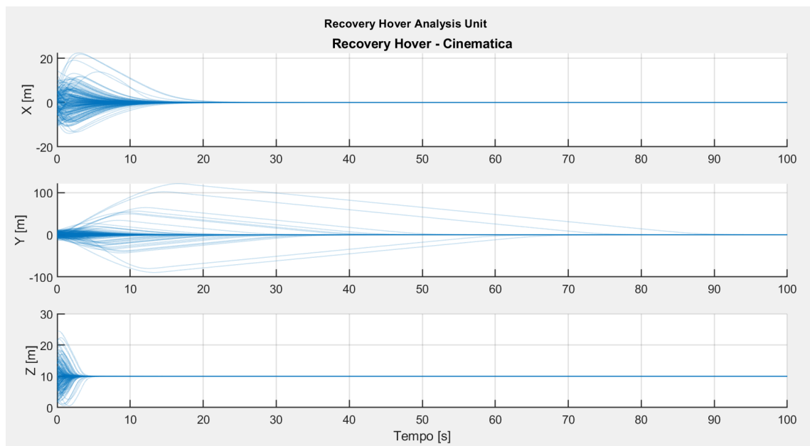
Figura 9.8: Evoluzione delle posizioni in hovering.
