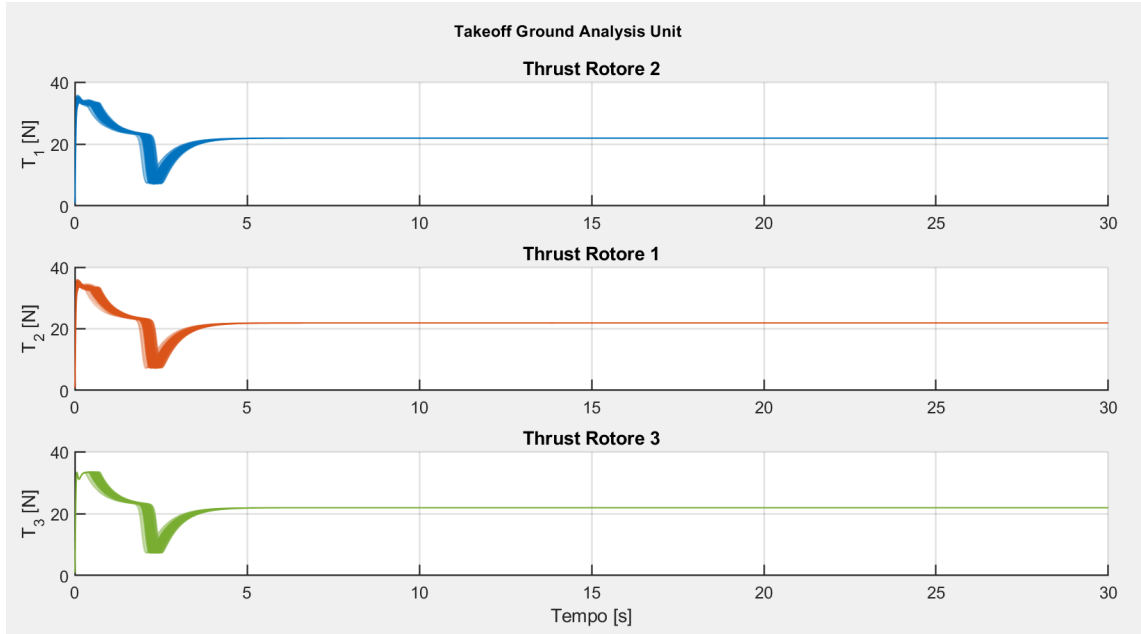
Figura 9.7: Evoluzione del thrust generato dai rotori durante il takeoff.
