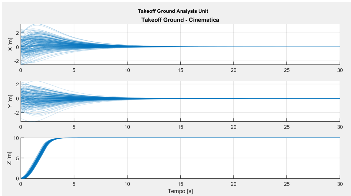
Figura 9.2: Evoluzione delle posizioni durante il takeoff.
