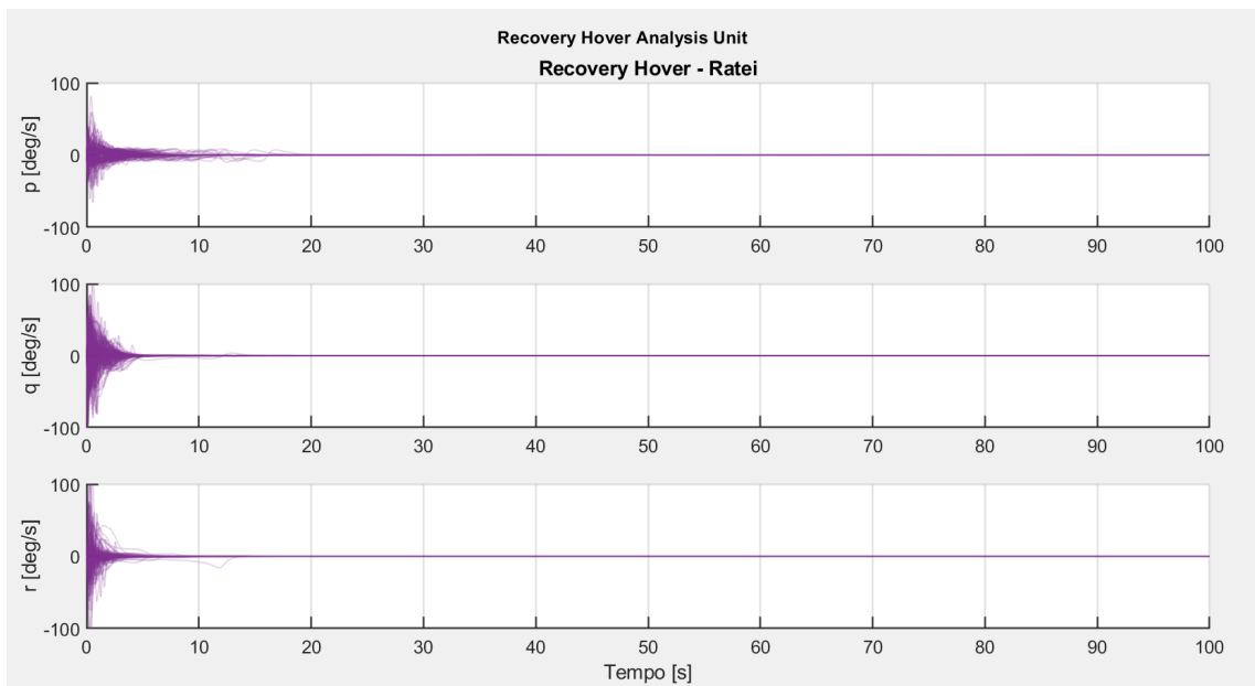
Figura 9.11: Evoluzione delle velocità angolari in hovering.
