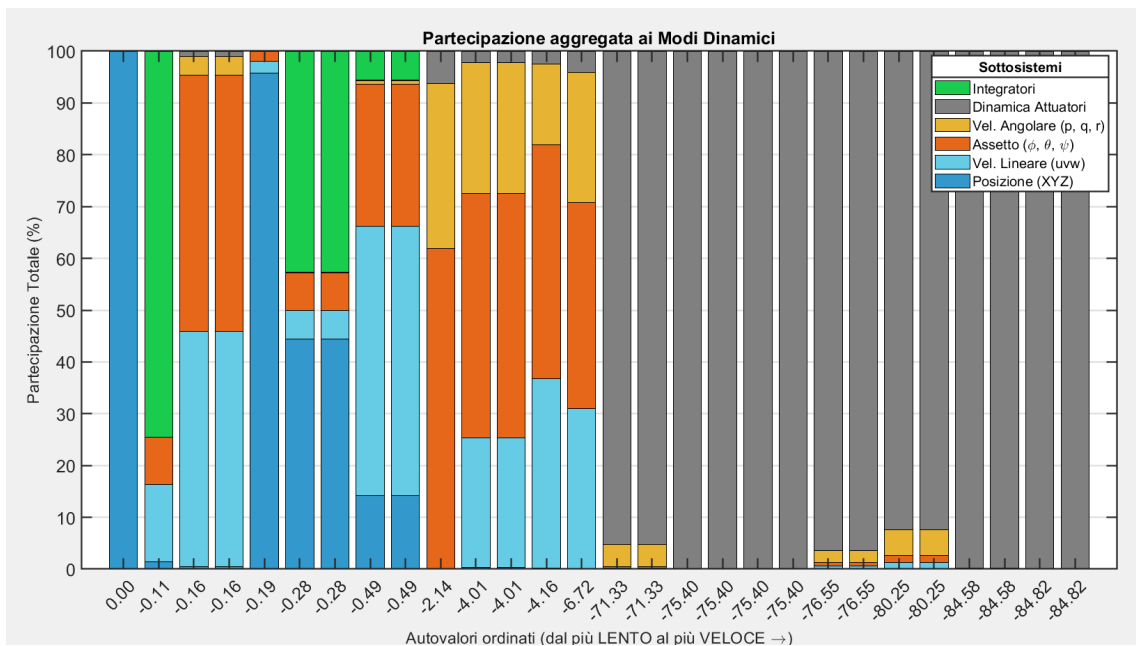
Figura 8.2: Analisi della partecipazione aggregata ai modi dinamici in crociera.
