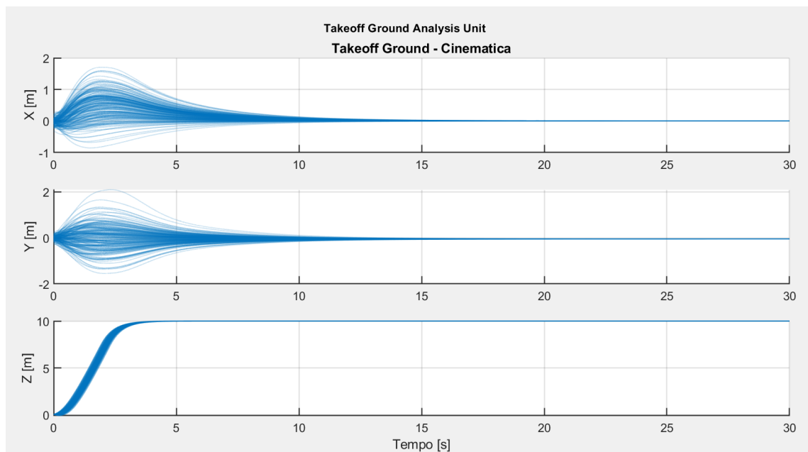
Figura 9.1: Evoluzione delle posizioni durante il takeoff.
