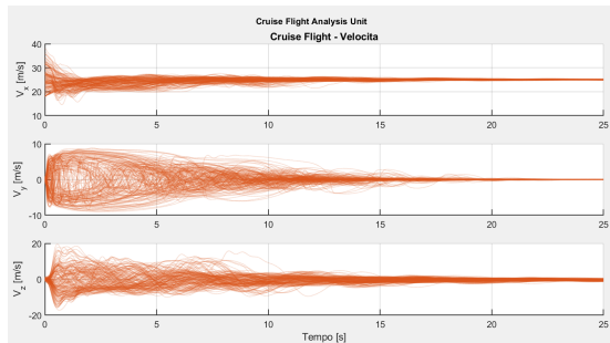
Figura 22: Velocità lineari in fase di crociera.
