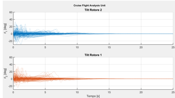
Figura 24: Angoli di Tilt
