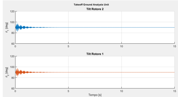
Figura 16: Angoli di Tilt
