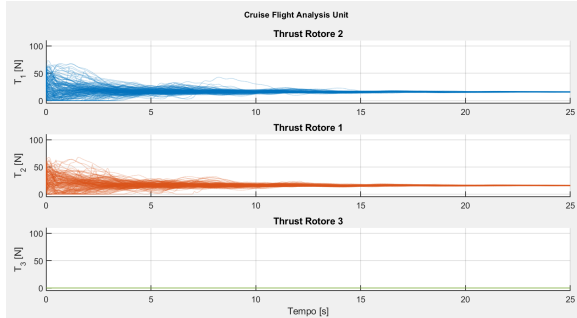
Figura 23: Spinta Rotori
