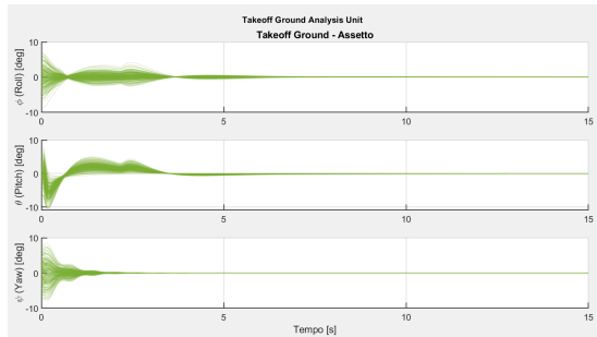
Figura 14: Angoli di Eulero.
