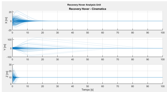
Figura 17: Posizioni in hovering.
