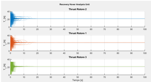
Figura 19: Spinta Rotori
