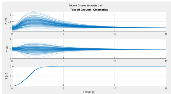
Figura 13: Posizioni durante il decollo.
