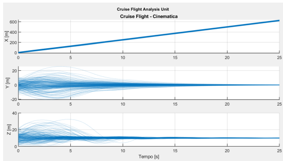
Figura 21: Posizioni in fase di crociera.
