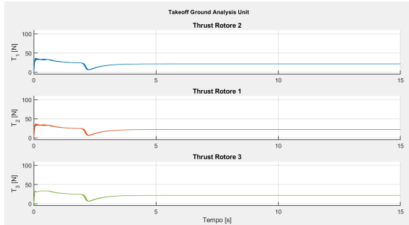
Figura 15: Spinta Rotori
