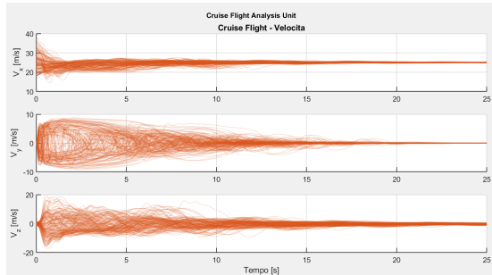
Figura 21: Velocità lineari in fase di crociera.
