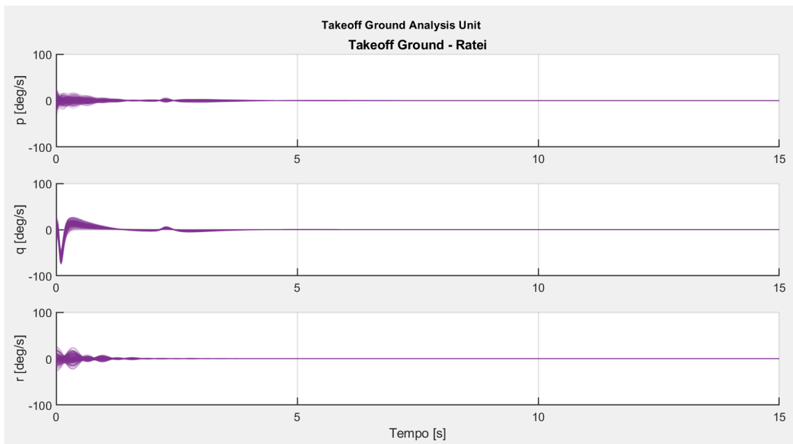
Figura 8.4: Evoluzione delle velocità angolari durante il takeoff.
