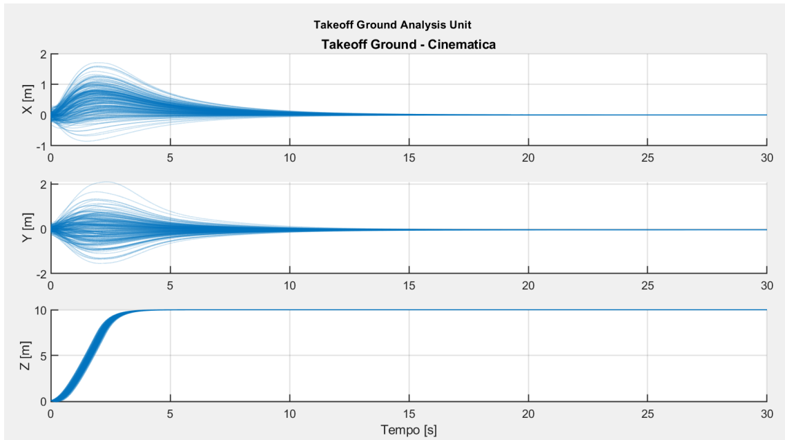
Figura 8.1: Evoluzione delle posizioni durante il takeoff.
