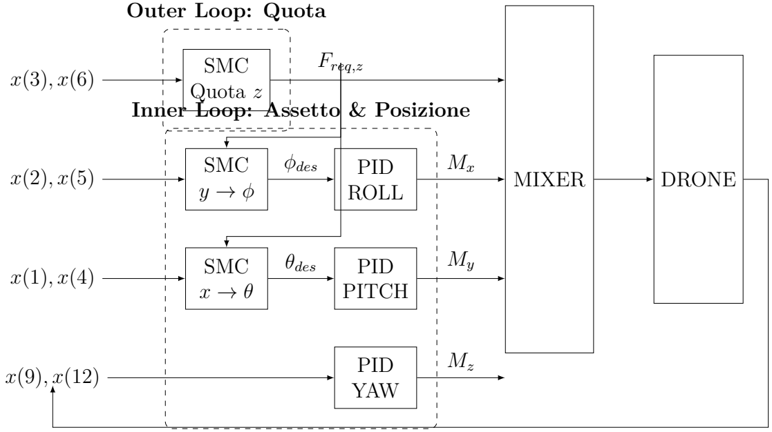
Figura 5.1: Schema a blocchi del controllo. L'SMC di quota fornisce la spinta totale F_{req,z} necessaria per le formule di inversione nel controllo planare.
