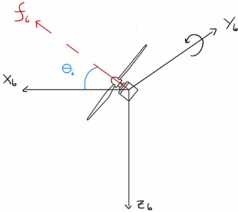
Figura 3.2: Tilt rotori anteriori ( X_b, Z_b ) Figura 3.3: Tilt rotore coda ( X_b, Y_b, Z_b )
