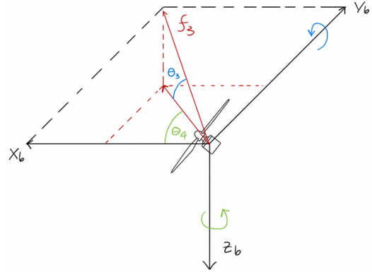
Figura 3.2: Tilt rotori anteriori ( X_b, Z_b ) Figura 3.3: Tilt rotore coda ( X_b, Y_b, Z_b )
