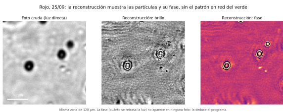
Rojo, 25/09, set 3: foto cruda, amplitud y fase reconstruidas de la misma zona de 128 µm.
