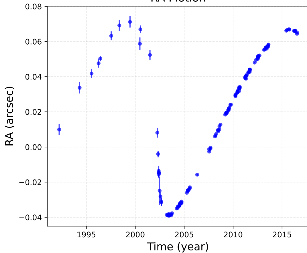
RA Motion
