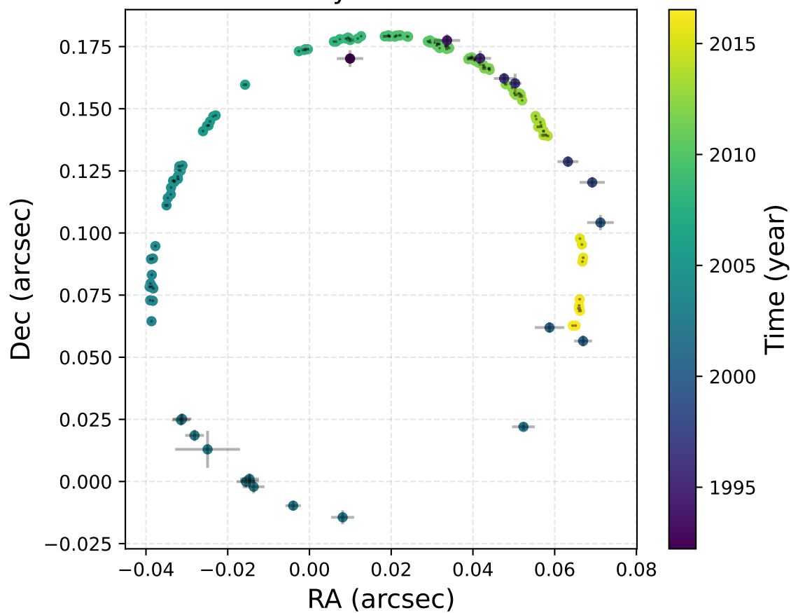
RA Motion
