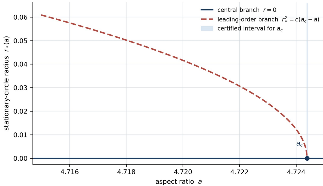
図1 局所分岐図。中心枝 r=0 は全軸比で存在する。 Q(a) \approx Q'(a_c)(a-a_c) より、破線は認証済み参照係数 c=6Q'(a_c)/H_4(a_c) \approx 0.39474123 を用いた主項 r_*(a)^2=c(a_c-a) であり、実測枝または大域的数値追跡ではない。淡青帯は a_c \in (4.72438, 4.72439) の認証区間を示す。
