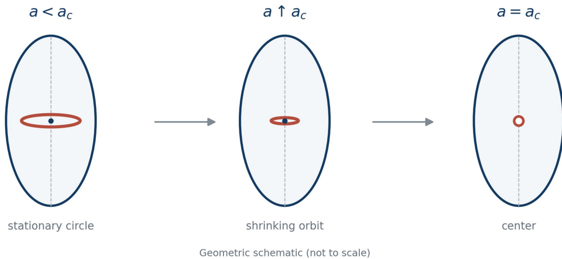
図2 停留円の中心への収縮を示す幾何学的模式図。赤線は赤道面内の停留円、青点は中心を表す。 a \uparrow a_c に伴って軌道半径は零へ近づき、臨界値で中心に合流する。形状・半径・軸比は説明のための模式表現であり、縮尺には従わない。
