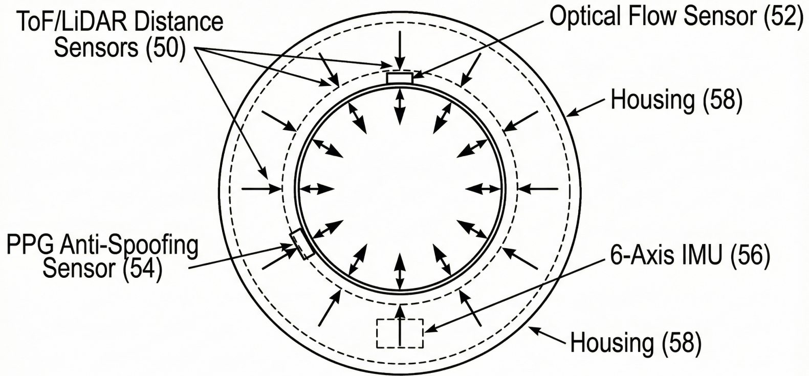
FIG. 3 - NODE 3
