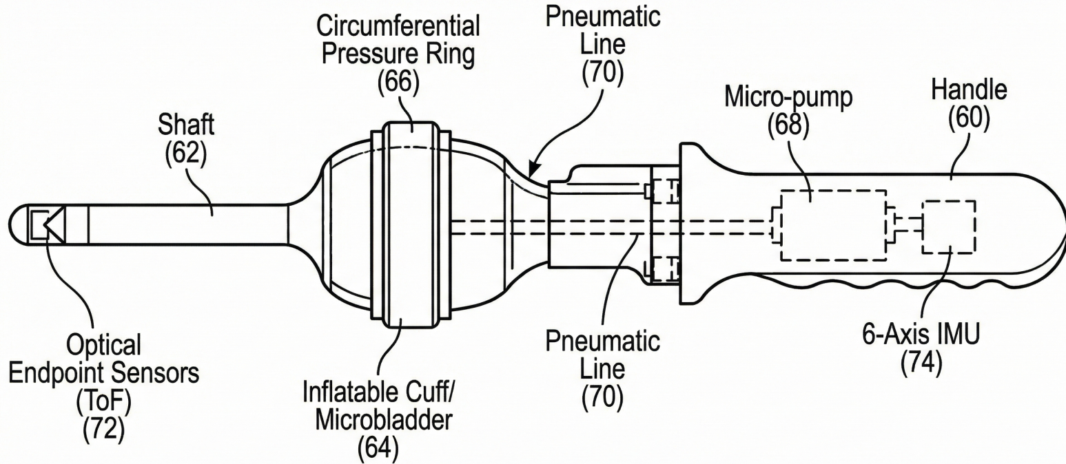
FIG. 4 - NODE 4
