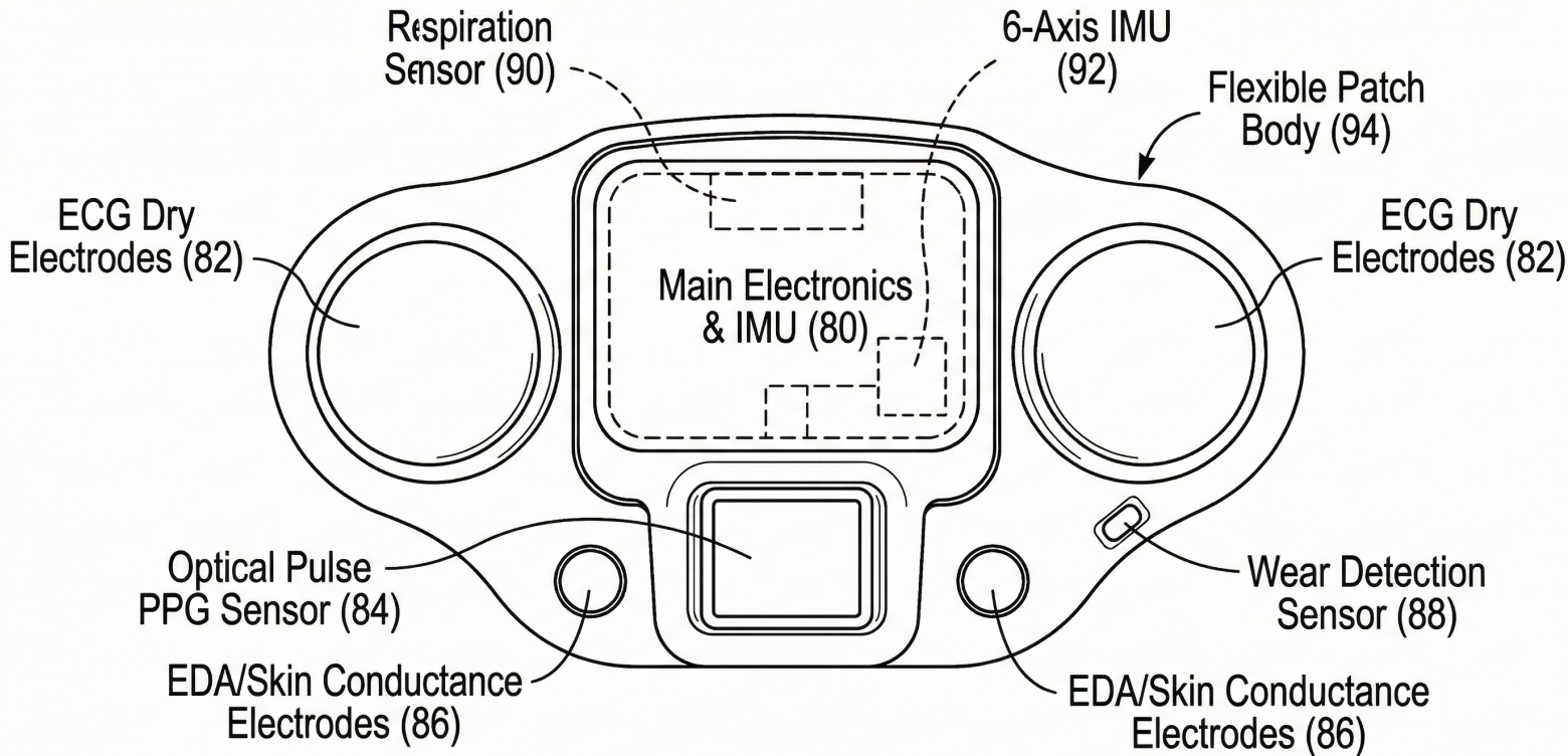
FIG. 5 - NODE 5
