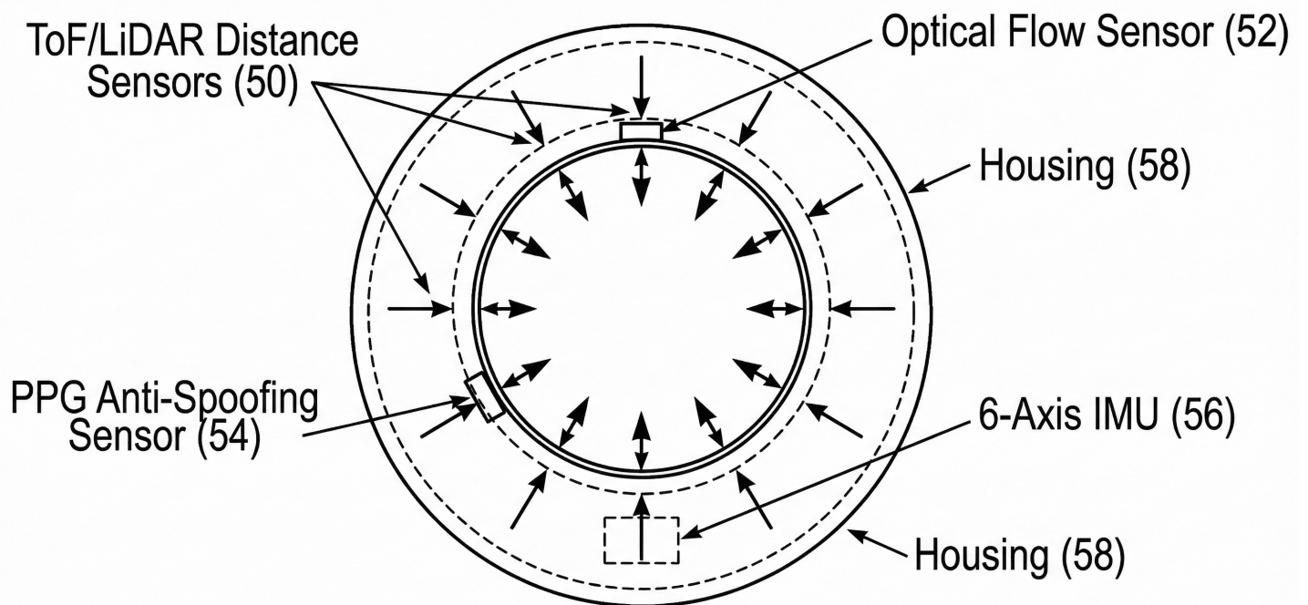
FIG. 3 - NODE 3
