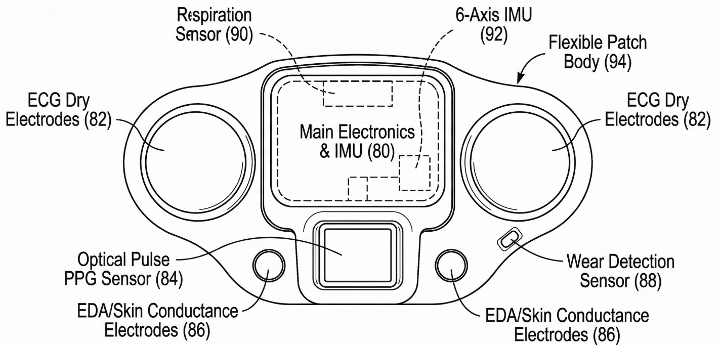
FIG. 5 - NODE 5
