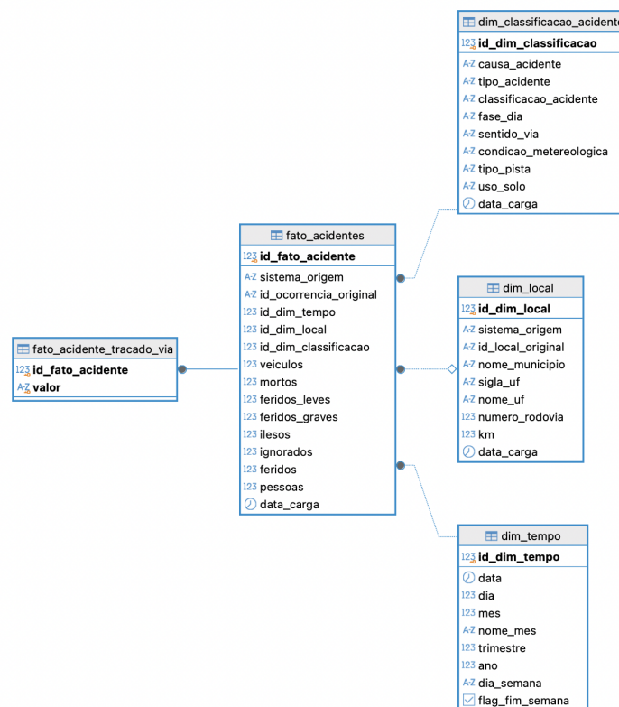
Figura 2 – Diagrama entidade-relacionamento do Data Mart em estrela
