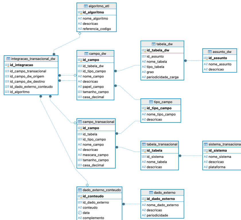
Figura 3 – Diagrama entidade-relacionamento do catálogo de metadados
