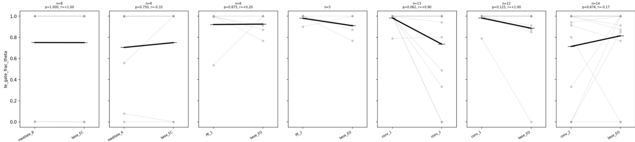
te_gate_frac_theta
