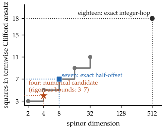
(d) termwise-Clifford price: integer 18 \rightarrow 512 half-offset 7 \rightarrow \text{dim } 8 ; four is numerical
