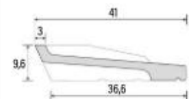
Appui carré R 410
