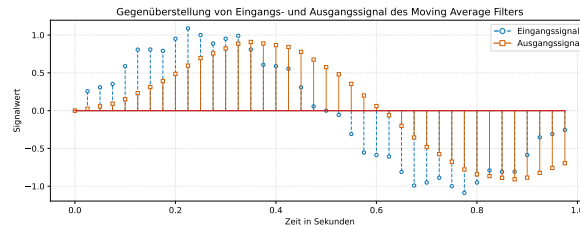
Abbildung 3.2: Das gefilterte Signal, über das ungefilterte Signal aus Abbildung 3.1 vorgeblendet
