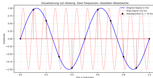
Abbildungung 2.2: Neben den beiden abgebildeten Kurven könnten unendlich viele weitere Kurven über die Abtastwerte gelegt werden
