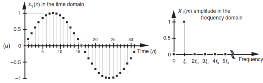
Abbildung 2.1: Links: Zeitdomäne eines Signals, Rechts: Frequenzdomäne desselben Signals [Lyo11, Kap. 1, S. 6]
