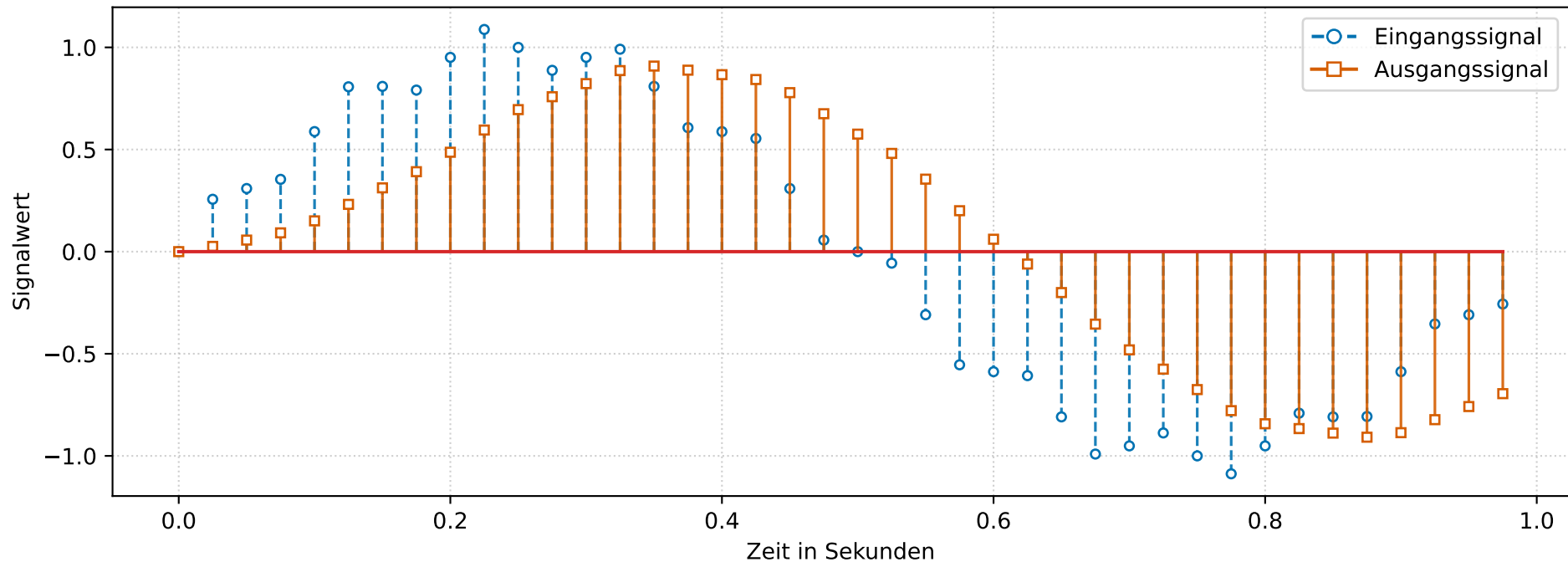
Gegenüberstellung von Eingangs- und Ausgangssignal des Moving Average Filters
