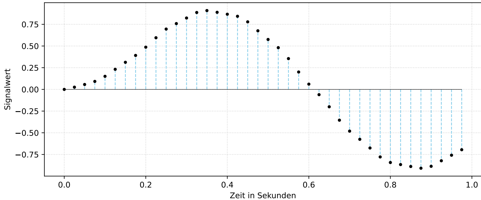
Zusammengesetzter Sinus nach Anwendung des Moving Average Filters
