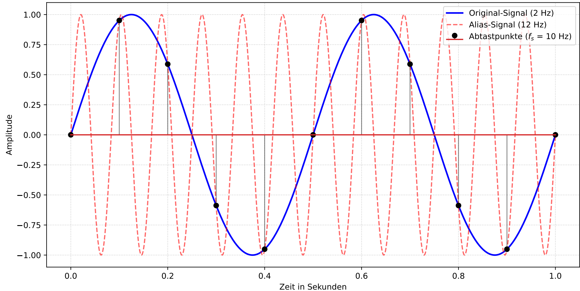
Visualisierung von Aliasing: Zwei Frequenzen, dieselben Abtastwerte
