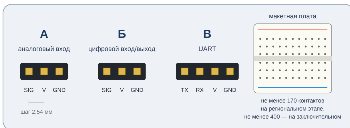
Рис. 6. Разъемы А, Б, В и макетная плата (схематично): шаг контактов 2,54 мм, порядок контактов — слева направо, как на рисунке
