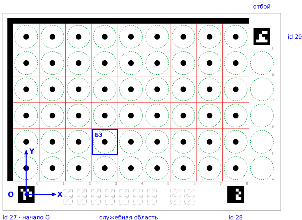
Рис. 2. Операционное поле: метки ArUco, оси координат и обозначение клеток (выделена клетка Б3: X = 84 мм, Y = 56 мм)
