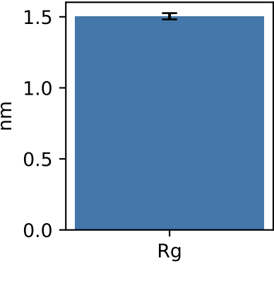
7. Rg
