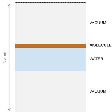
\beta -Casein slab
