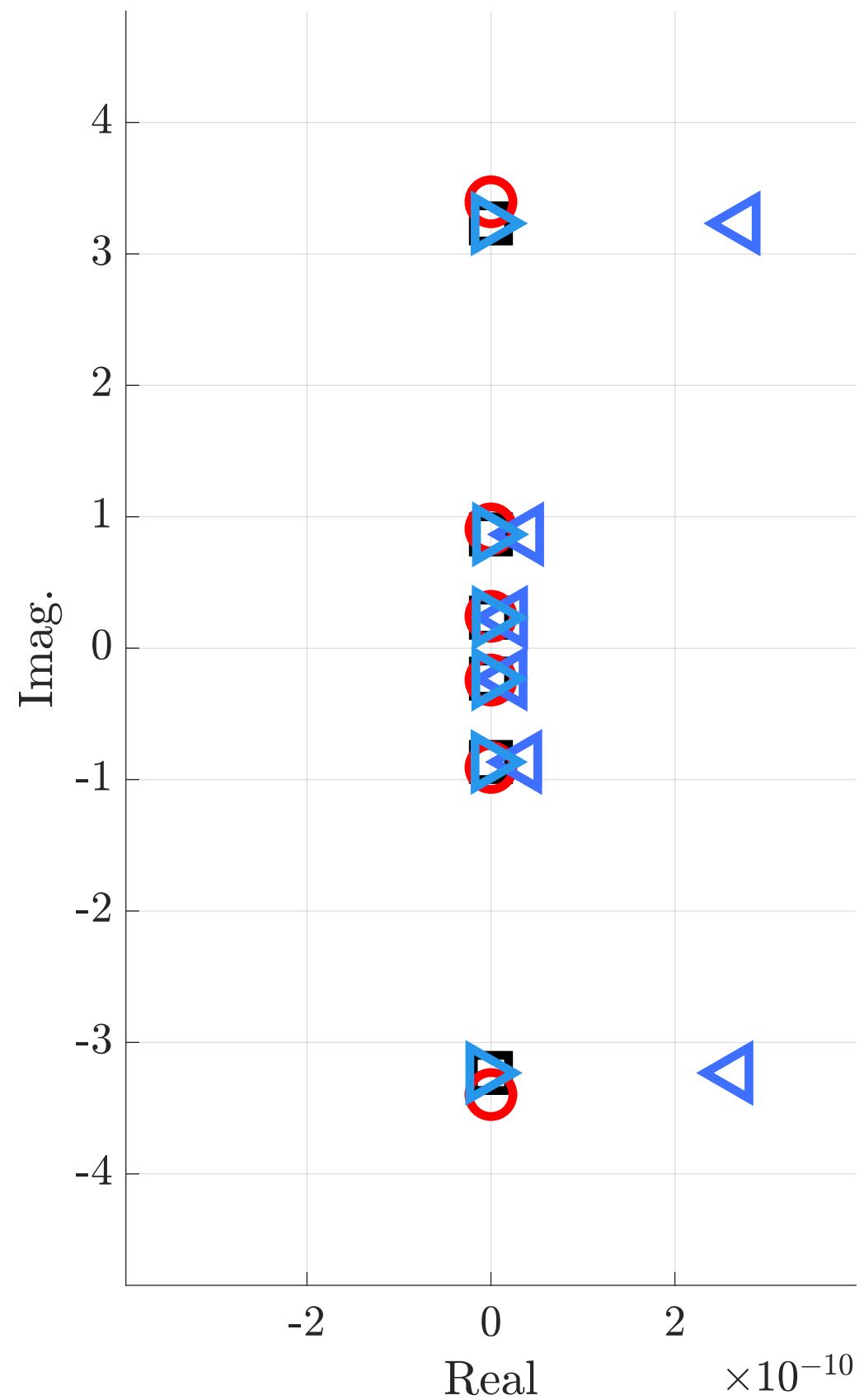
Poles
