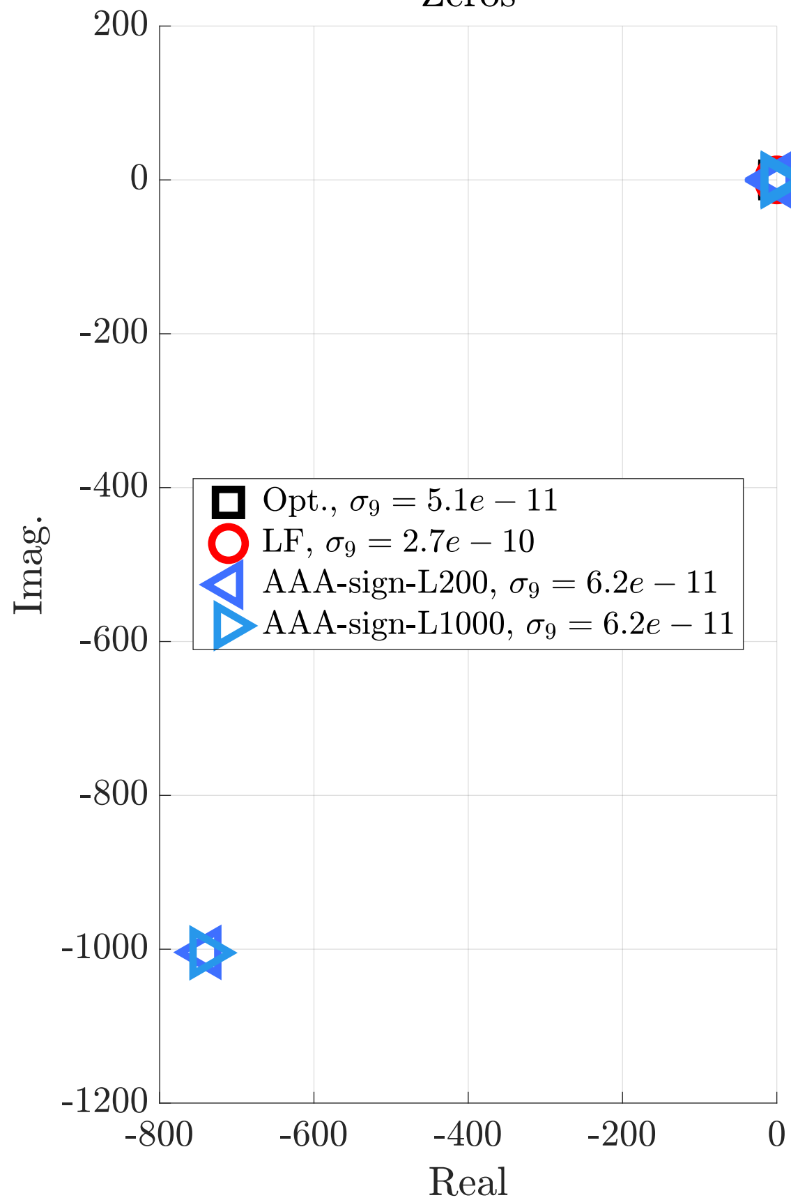
Zeros
