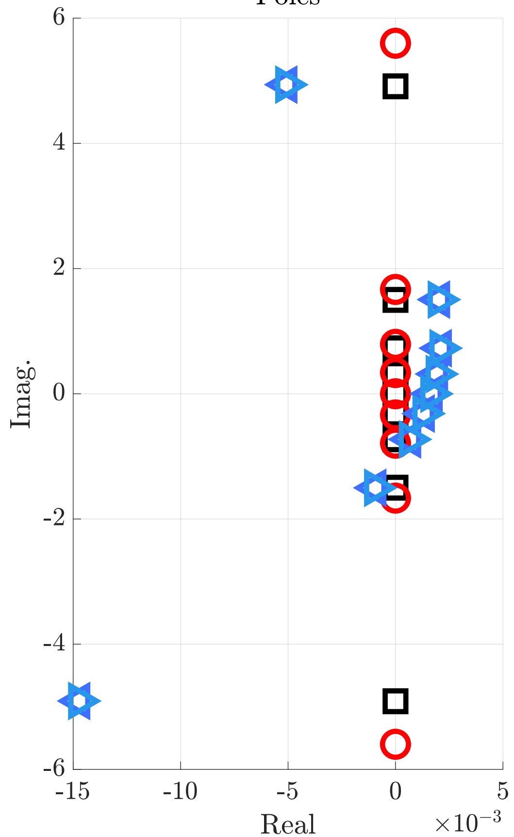
Poles
