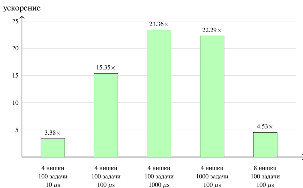
Фигура 6. Относително ускорение на асинхронната пропускливост спрямо синхронната
