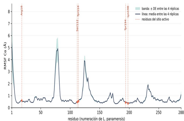
Figura 2. PTR1: flexibilidad Cα por residuo (RMSF) tras descartar los primeros 10 ns. Línea: media de las cuatro cadenas dentro de cada una de cuatro réplicas independientes; banda: desviación estándar entre réplicas. Las marcas en rojo señalan los residuos del sitio activo, que caen en zonas de baja flexibilidad.
