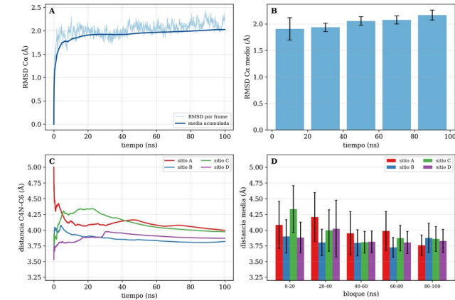
Figura 2. PTR1: estabilización de las métricas durante la producción de 100 ns. (A) RMSD Cα global por frame y su media acumulada; (B) RMSD Cα medio por bloques de 20 ns; (C) distancia catalítica C4N–C6 (media acumulada) en los cuatro sitios; (D) la misma distancia por bloques de 20 ns. Las medidas se asientan tras un breve ajuste inicial y luego se mantienen estables (variación menor a 0.30 Å).
