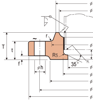
C TYPE : NOMINAL SIZE 65A-250A
