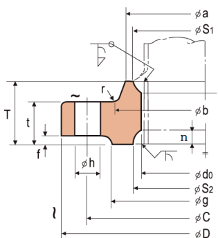
B TYPE : NOMINAL SIZE 10A-50A
