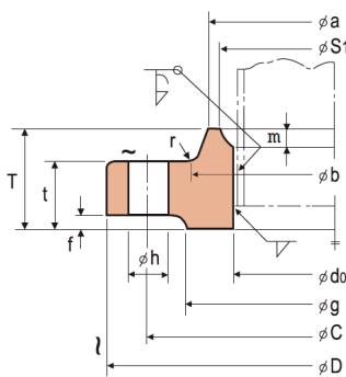
A TYPE : NOMINAL SIZE 10A-250A
