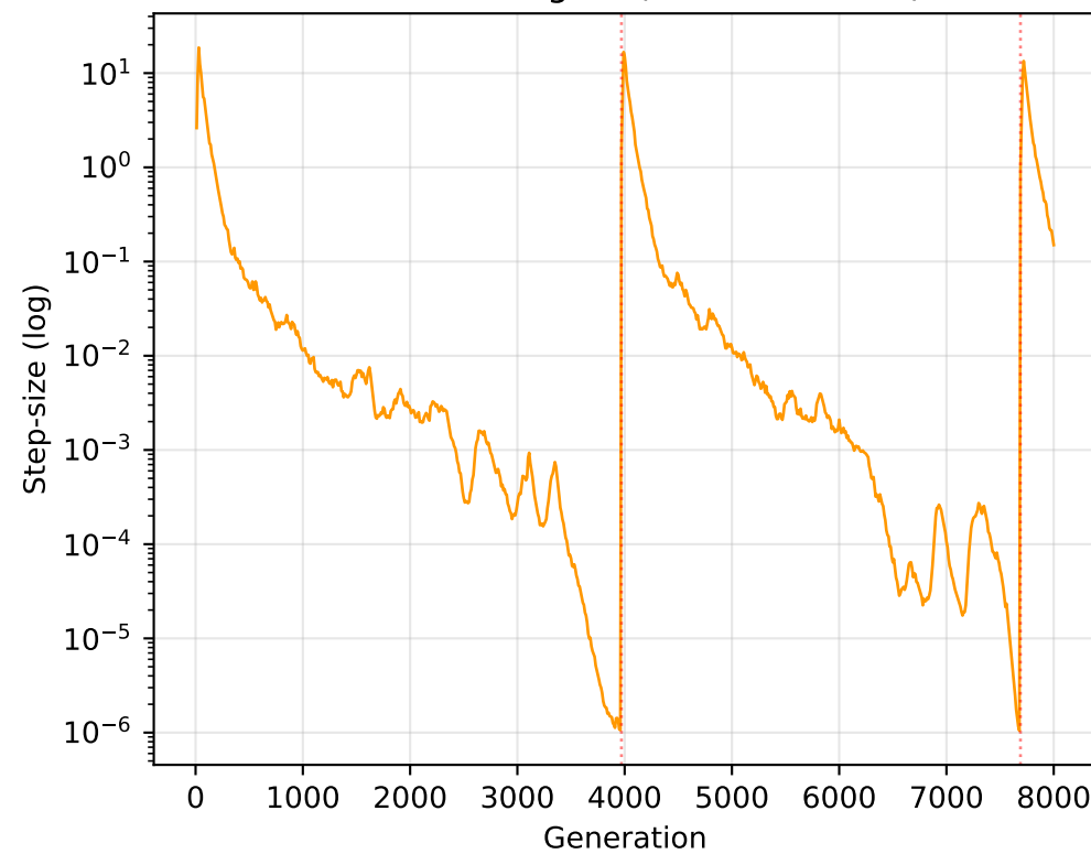
E. CMA-ES sigma (restarts visible)
