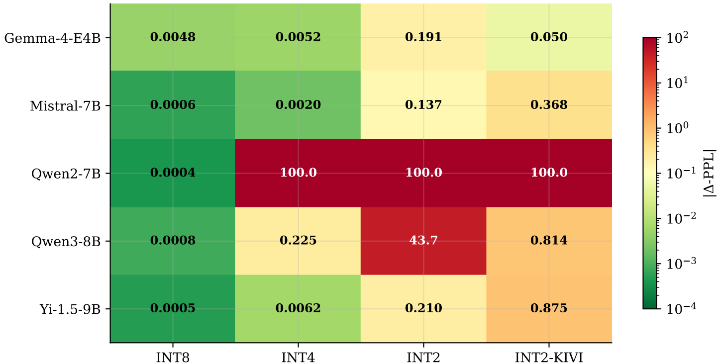
|\Delta\text{-PPL}| Heatmap (höchste Kontextlänge je Modell, WikiText-2) Grün = verlustfrei, Rot = starke Degradation (log scale)
