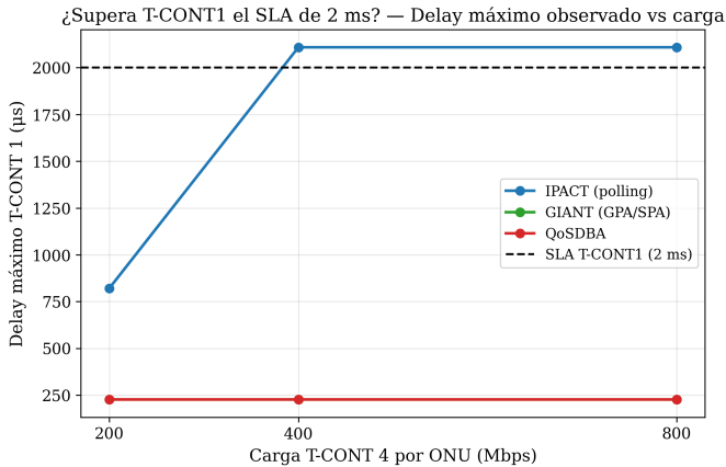
Figura 5. Delay máximo de T-CONT1 vs. carga, con cota de SLA (2 ms).
