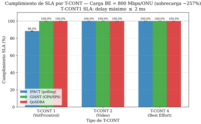
Figura 4. Cumplimiento de SLA por T-CONT a 800 Mbps/ONU.
