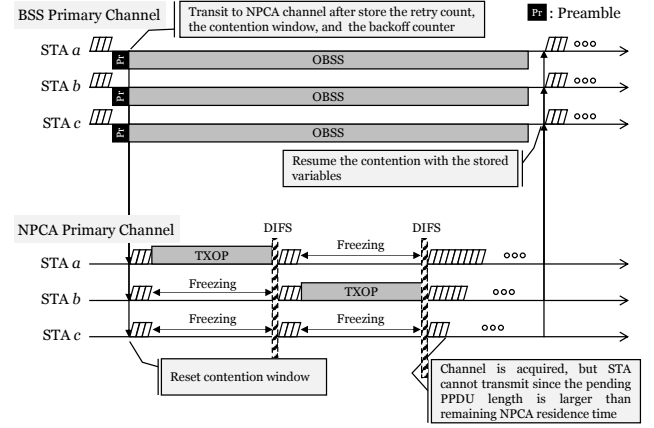
(a) NPCA baseline (BEB).
