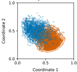
Epoch 10
