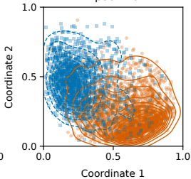
Epoch 20
