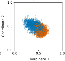
Epoch 5
