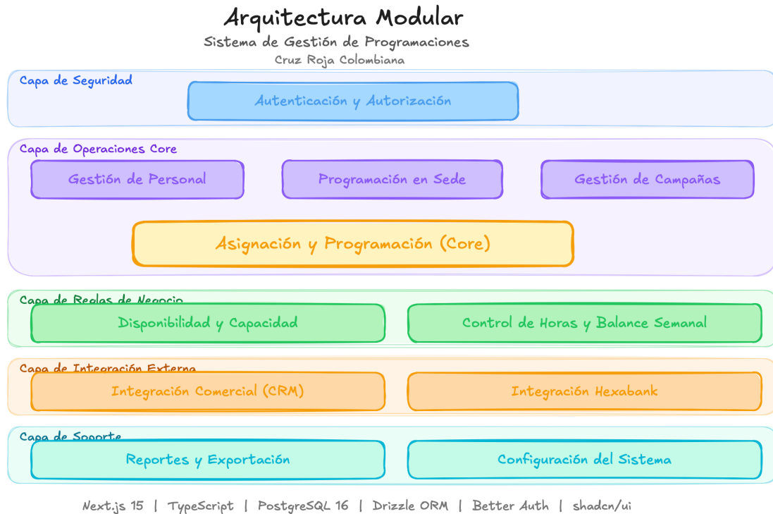
Figura 6: Arquitectura del sistema: módulos principales organizados por función
