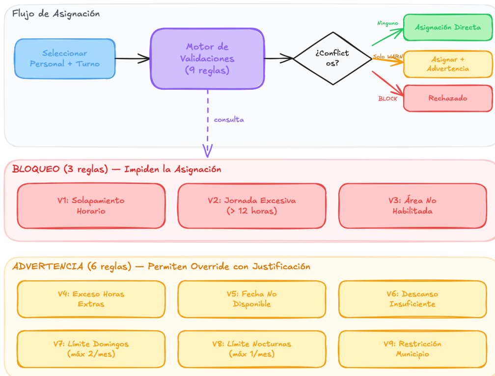
Figura 3: Flujo de asignación inteligente: motor de 9 validaciones
