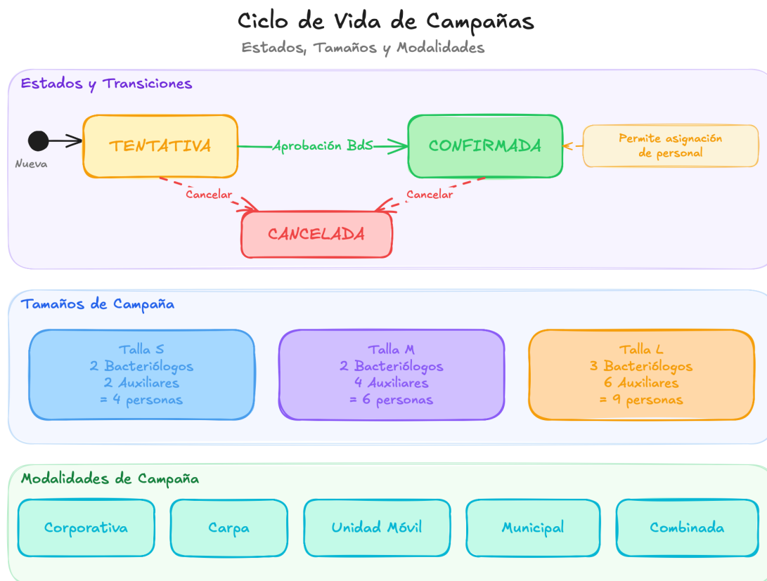
Figura 1: Ciclo de vida de campañas: estados, transiciones, tamaños y modalidades
