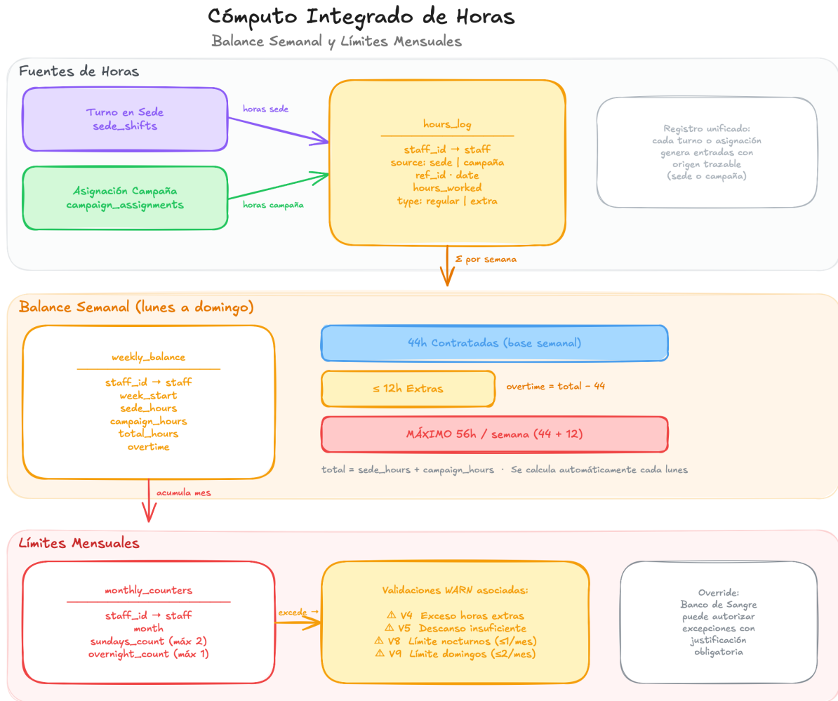
Figura 2: Cómputo integrado de horas: balance semanal (44h + 12h extras) y límites mensuales
