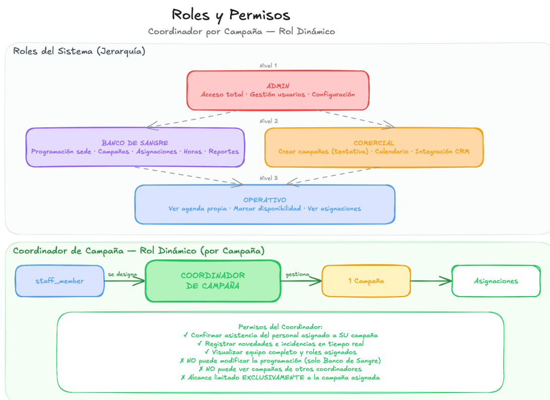
Figura 5: Jerarquía de roles del sistema + coordinador de campaña (designación dinámica)
