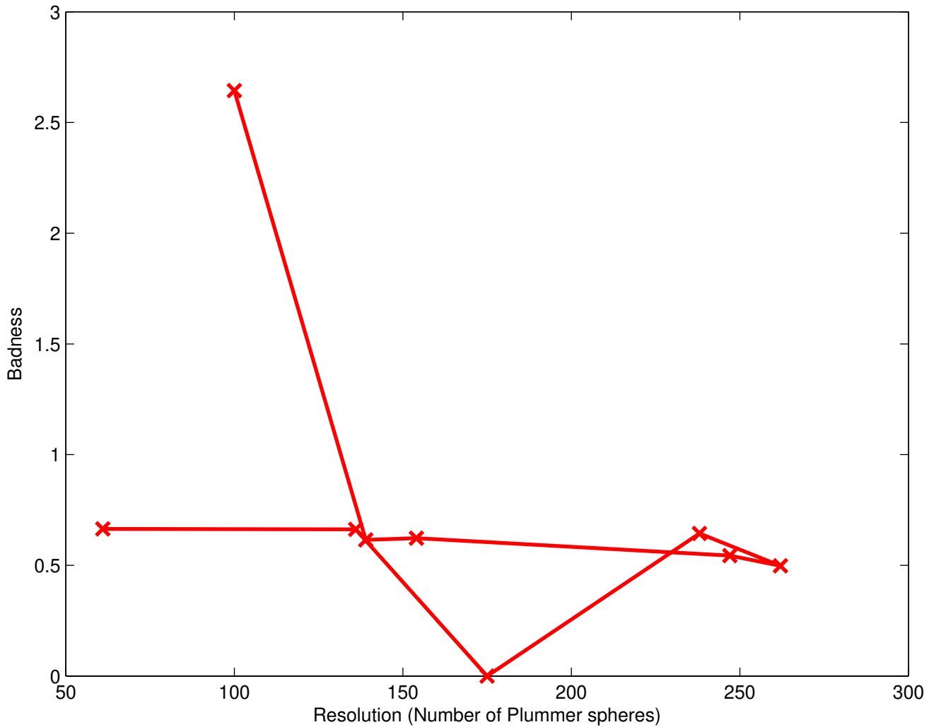
Abell 3827
