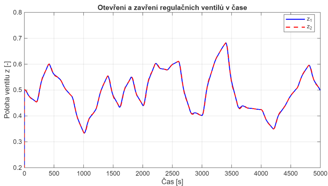
Obrázek 18: Akční zásahy ventilů z_1, z_2 při extrémním stochastickém zarušení
