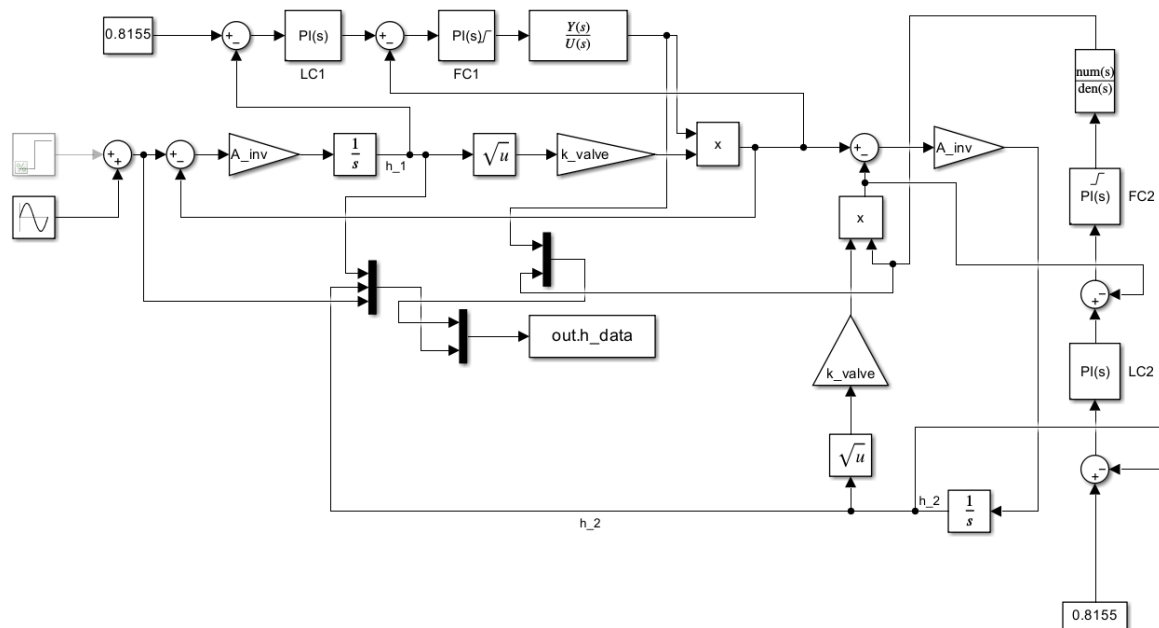
Obrázek 11: Simulink model kaskádního řízení nádrží
