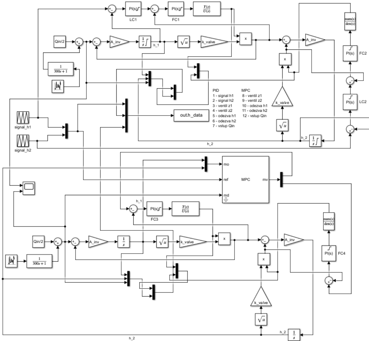
Obrázek 20: Komplexní simulační schéma pro přímé porovnání PID a MPC regulace v identických podmínkách
