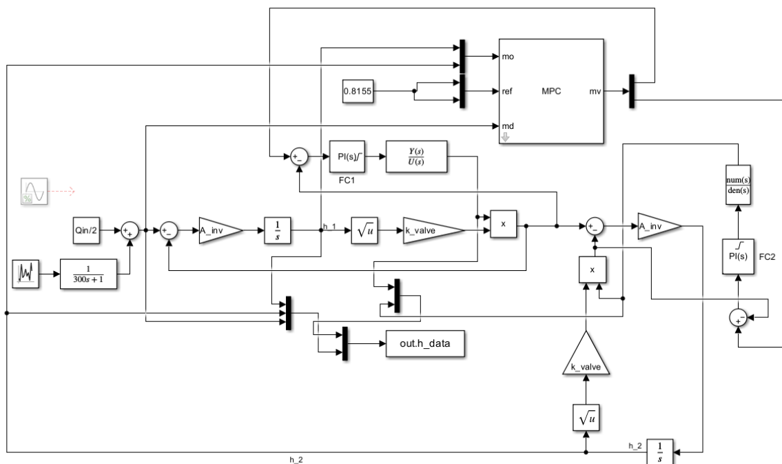
Obrázek 17: Simulink model se stochastickým zarušením vstupního průtoku (Úkol 6)
