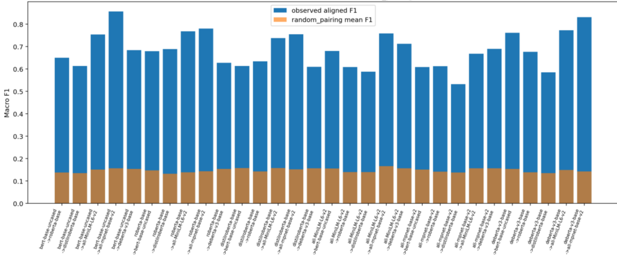
UPAT Procrustes null baseline: random_pairing
