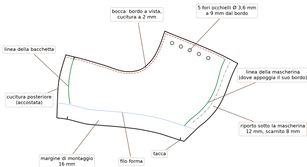
Figura 7. Il cartamodello del quartiere esterno con i suoi segni.
