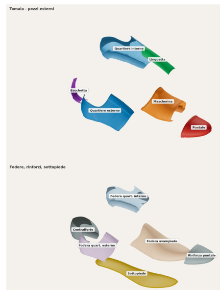
Figura 3. Esploso: sopra i pezzi esterni della tomaia, sotto fodere, rinforzi e sottopiede.
