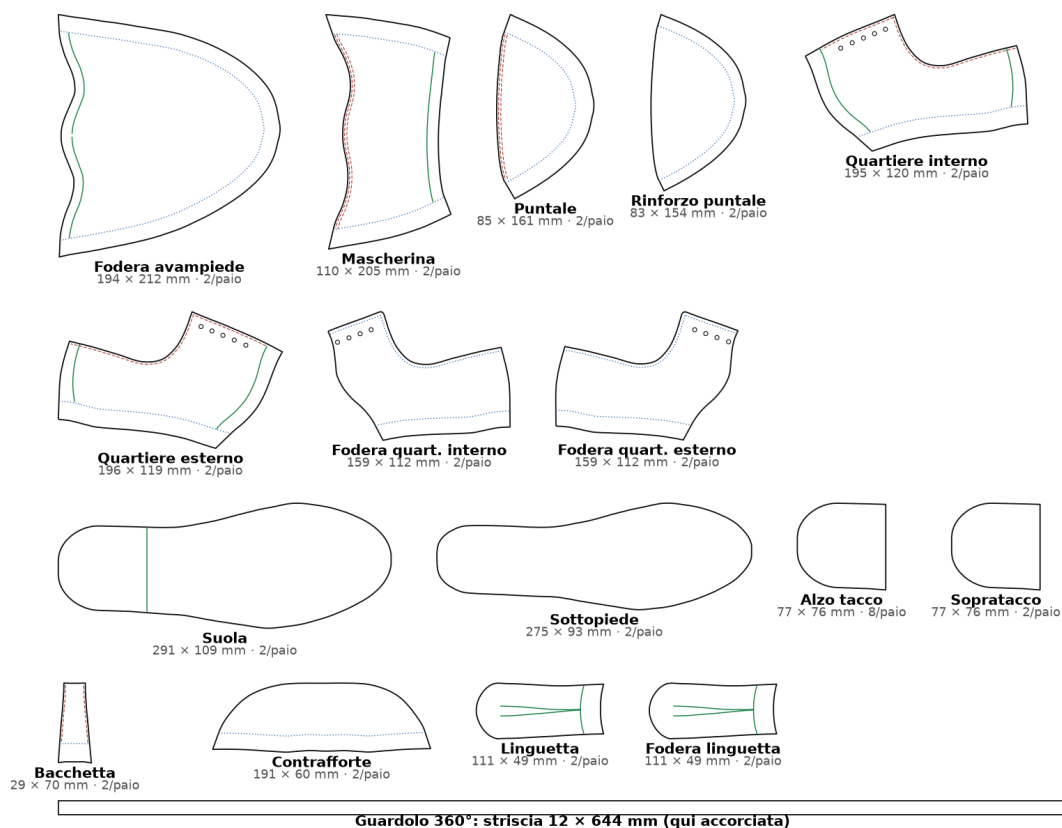
Figura 9. Tutti i cartamodelli alla stessa scala (ridotta). Il guardolo è accorciato.
