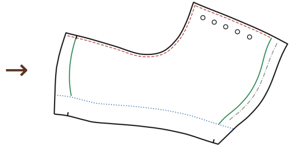
Figura 4. Il quartiere esterno sulla forma (in blu) e lo stesso pezzo steso in piano, con margini e segni.
