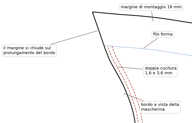
Figura 6. Angolo della mascherina tra bordo a vista e margine di montaggio.
