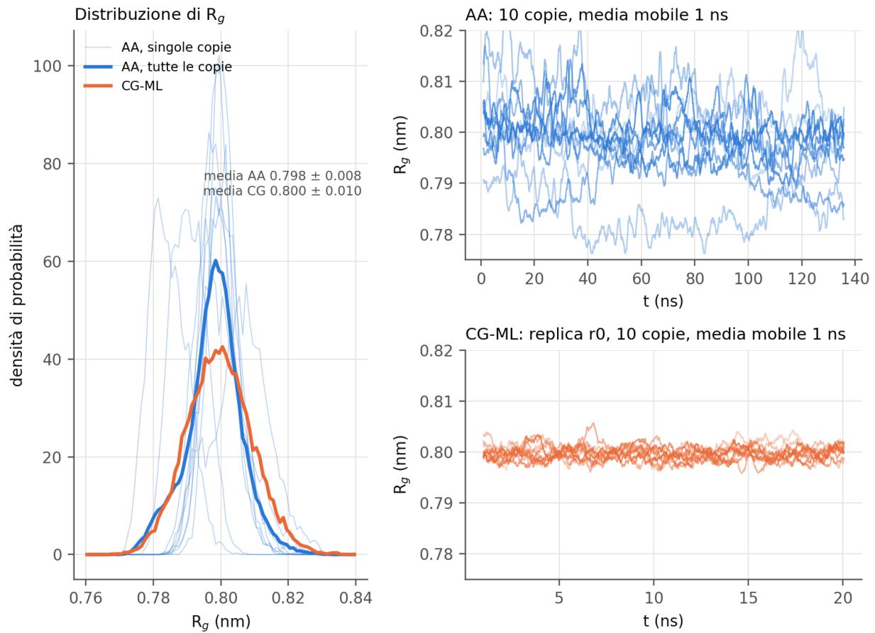
Figura 4. Sinistra: distribuzione di R_g (AA: singole copie in linea sottile, insieme in linea spessa; CG-ML: tutte le copie e replicas). Destra: serie temporali con media mobile di 1 ns, AA su 136 ns e CG-ML (replica r0) su 20 ns, stessa scala verticale.
