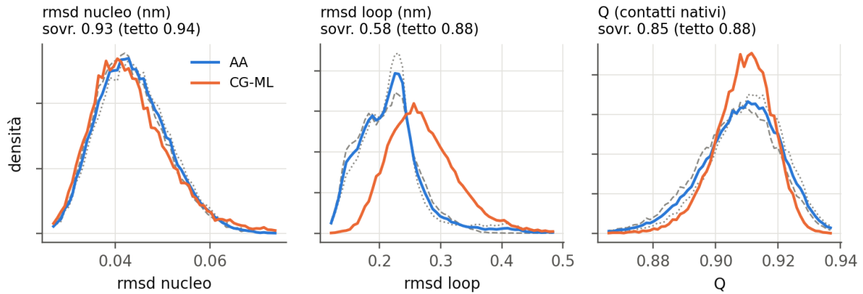
Figura 5. Distribuzioni di rmsd del nucleo, rmsd dei loop e frazione di contatti nativi Q (grigio: metà AA). Nei titoli la sovrapposizione CG-AA e il tetto.
