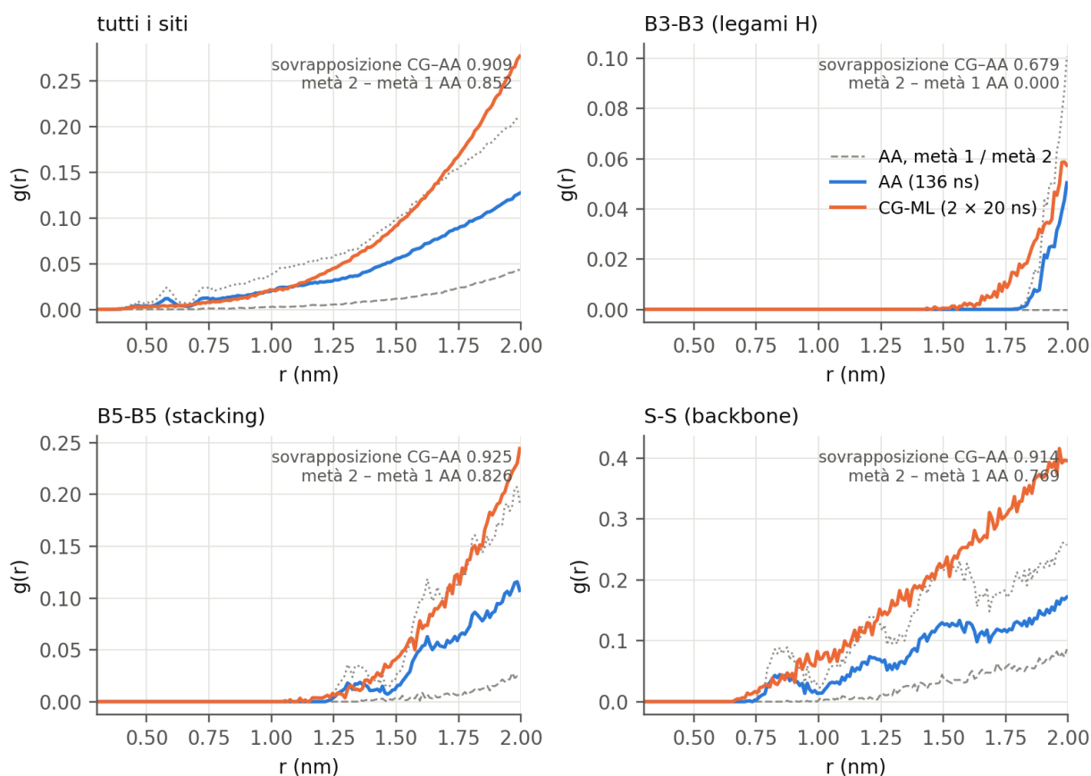
Figura 3. g(r) fra siti di copie diverse, stessi colori della figura 2. Le due metà AA differiscono di un fattore \sim 5 : gli incontri fra copie nell'AA sono pochi eventi lunghi.
