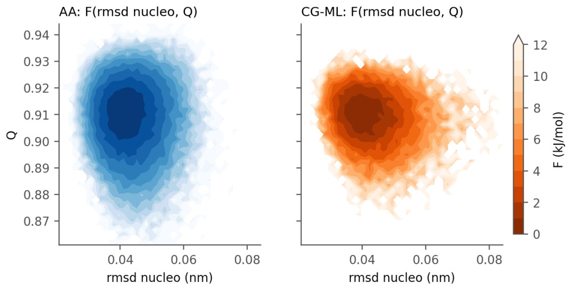
Figura 6. Energia libera F = -kT \ln p(rmsd\ nucleo, Q) , AA e CG-ML. La JSD fra le FES (script 46) è 0,0787, uguale al tetto AA contro sé stesso (0,0786); il CG è più rumoroso per il numero minore di frame (20 080 contro 67 880 copie-frame).
