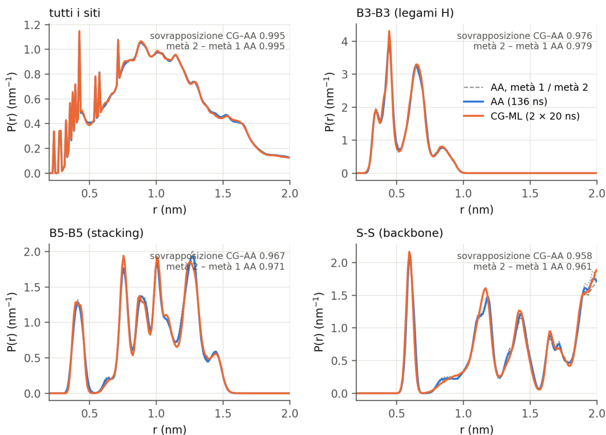
Figura 2. P(r) intramolecolari per canale. Blu: AA su 136 ns; arancione: CG-ML su 2 \times 20 ns; grigio tratteggiato e punteggiato: prima e seconda metà dell'AA. In alto a destra la sovrapposizione CG-AA e il tetto (metà 2 contro metà 1).
