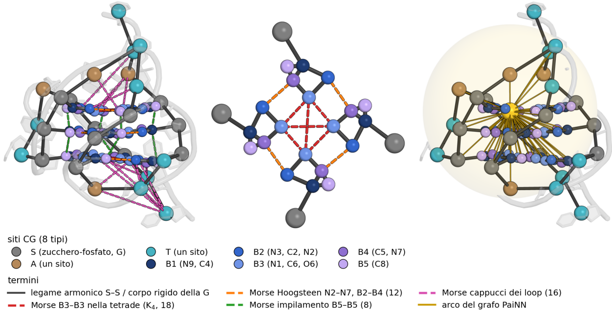
Figura 1. Il modello CG sulla struttura nativa 2JPZ (struttura di partenza delle simulazioni AA, mappata sui siti CG; in grigio trasparente il DNA atomistico). a : siti colorati per tipo; legami armonici del backbone e scheletro rigido delle guanine in grigio scuro; contatti Morse tratteggiati per classe. b : la tettrade 1 (G4, G12, G16, G22) vista lungo l'asse del quadruplex, con i sei Morse B3-B3 (lati e diagonali) e i quattro Morse di Hoogsteen B2-B4. c : il grafo su cui agisce PaiNN per il sito B3 di G16; la sfera ha raggio r_c = 1,26 nm e contiene 76 degli altri 85 siti della copia. Non sono disegnati angoli, diedri e WCA. Figura generata con PyMOL.
