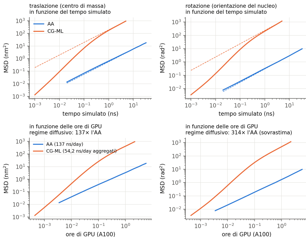
Figura 7. In alto: MSD in funzione del tempo simulato; tratteggiato 6Dt con D dal tratto lineare. In basso: le stesse curve in funzione delle ore di GPU A100 (AA 137 ns/day; CG-ML 54,2 ns/day aggregati su 2 replicas).
