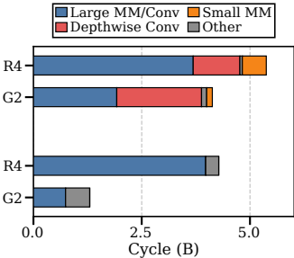
SqueezeNet MobileNetV2
