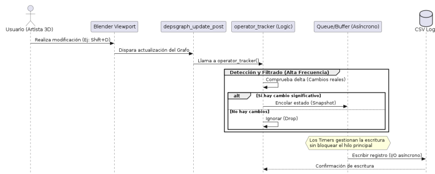
Figura A.1: Diagrama de flujo del sistema de captura y análisis planificado.
