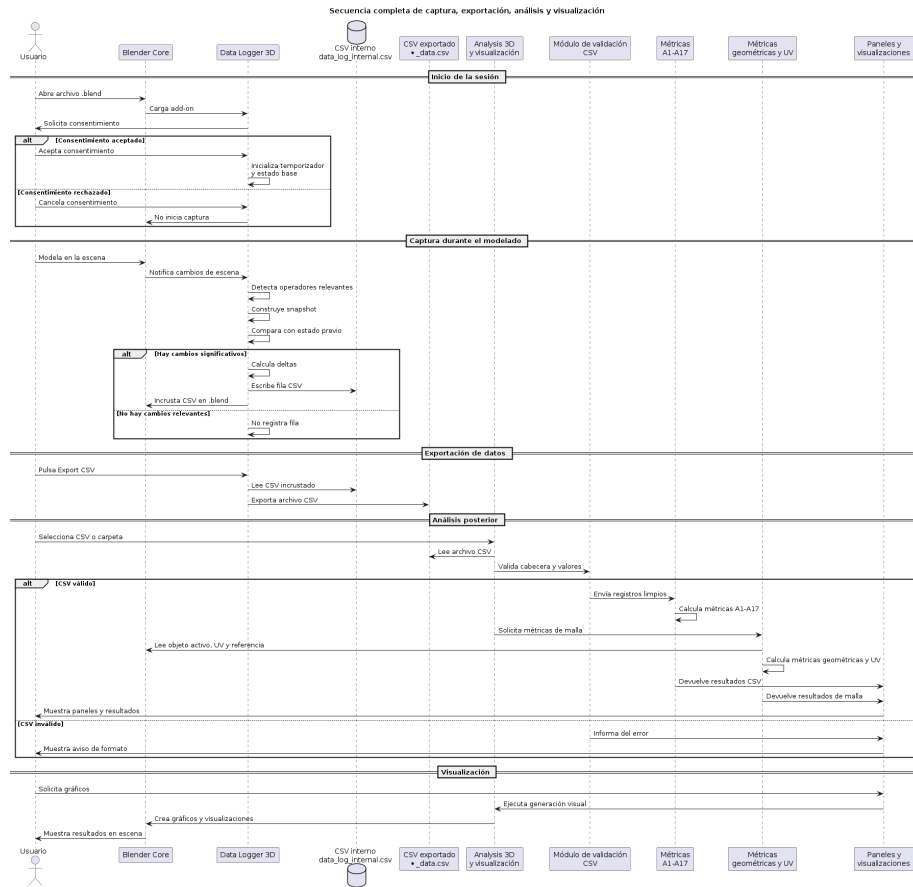
Figura C.4: Secuencia de interacción completa entre Blender, el add-on Data Logger 3D, el CSV intermedio y el add-on de análisis y visualización.
