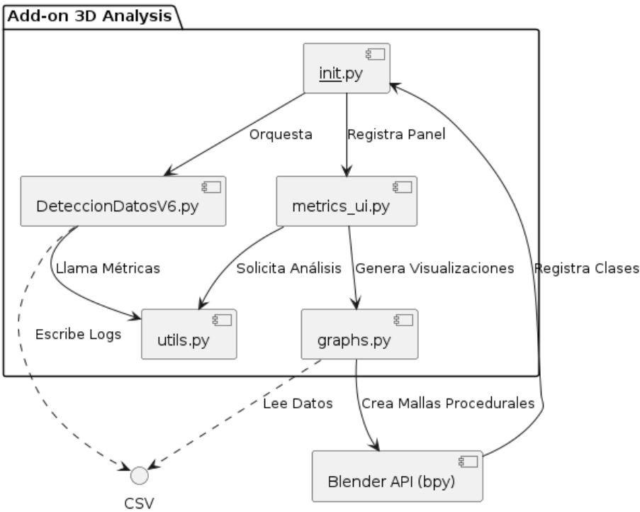
Figura C.2: Organización general de componentes y comunicación entre el logger, el CSV y el add-on de análisis.
