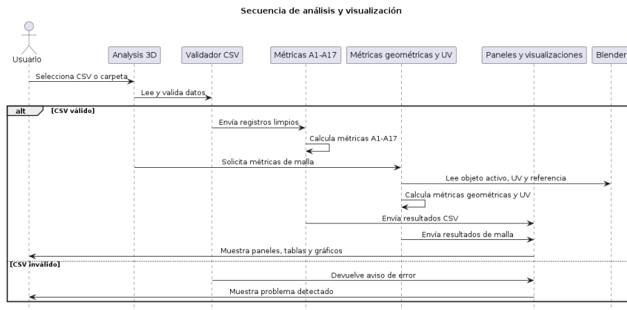
Figura C.7: Secuencia de análisis, cálculo de métricas y visualización de resultados en el segundo add-on.
