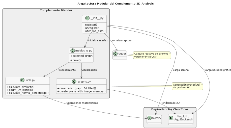
Figura C.3: Estructura modular del código y separación entre lógica de cálculo, interfaz y visualización.
