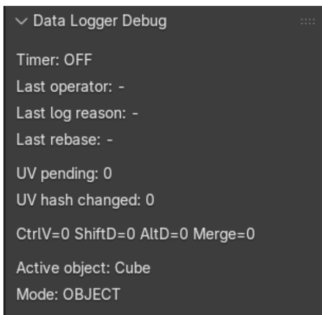
Figura D.2: Panel de depuración del add-on Data Logger 3D durante una sesión de captura.
