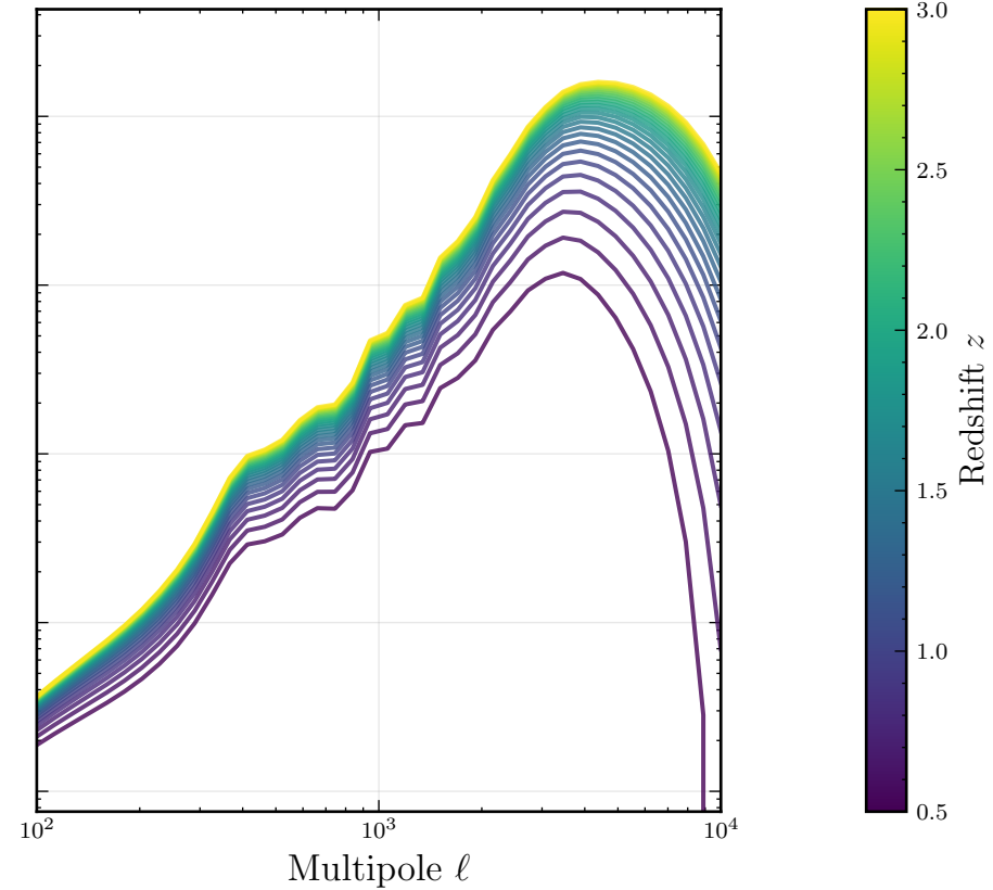
nDGP SNR
