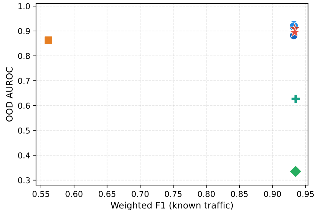
CTU-IoT-23
