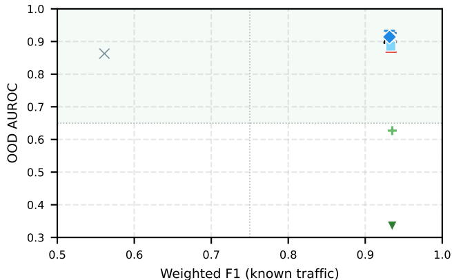
CTU-IoT-23
